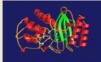
\beta -lactamase
